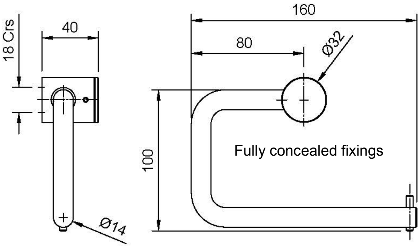
180° Pivoting arm
